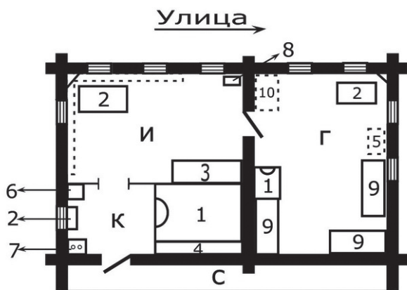
Рис. 2. План избы:
