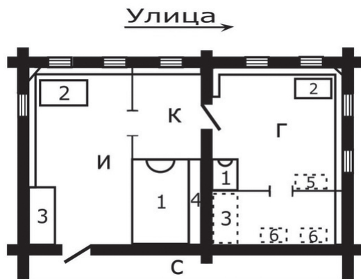
Рис. 1. План избы: И — изба, К — куть, Г — горница, С — сени; 1 — печь, 2 — стол, 3 — кровать, 4 — голбец (чулан), 5 — горка, 6 — сундук
