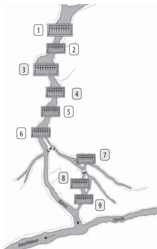
Рисунок 1. Схема Вахшского каскада ГЭС
