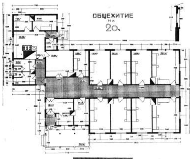
Илл.3. Общежитие (одноэтажное, каменное) на 20 человек. Проект. 1929.
