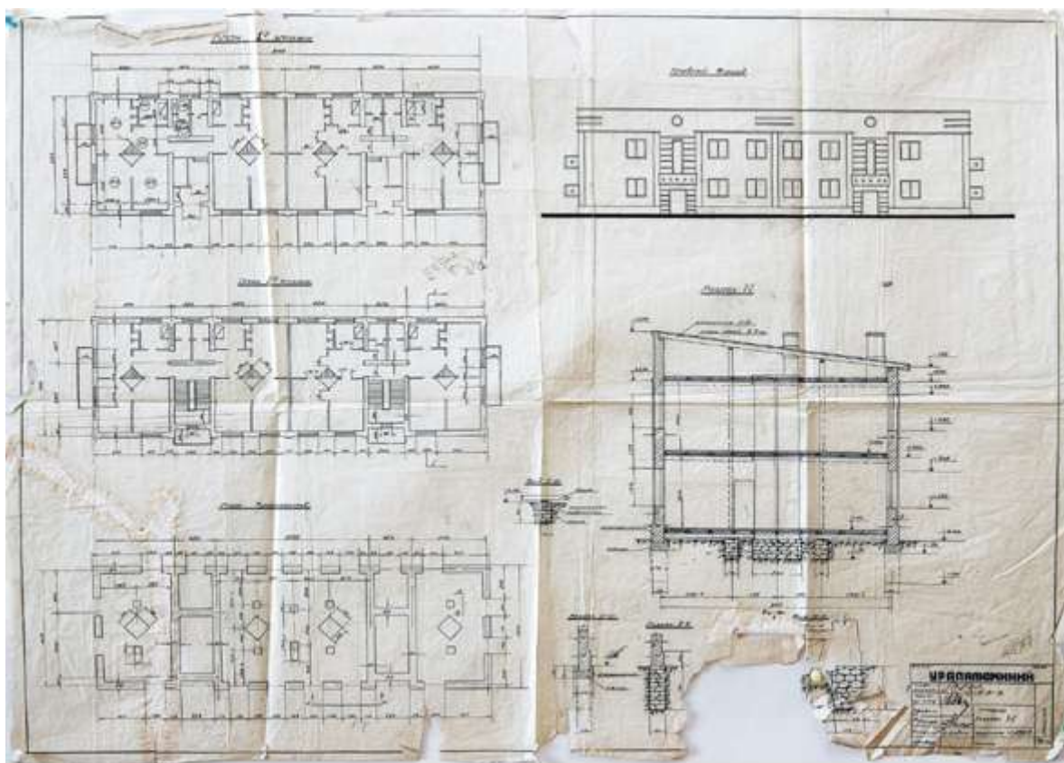
Илл.23. Проект брусково-каркасного жилого дома БК-8. "Уралалюминий" УАЗ, 1935 г. (Архив УАЗ-СУАЛ). Источник: Гаврилова С.И. Архитектура 1930-х годов Красногорского района г. Каменска-Уральского [Электронный ресурс] / С.И. Гаврилова //Архитектон: известия вузов. - 2009. -№3 (27). - Режим доступа: http://archvuz.ru/numbers/2009_3/ta1
