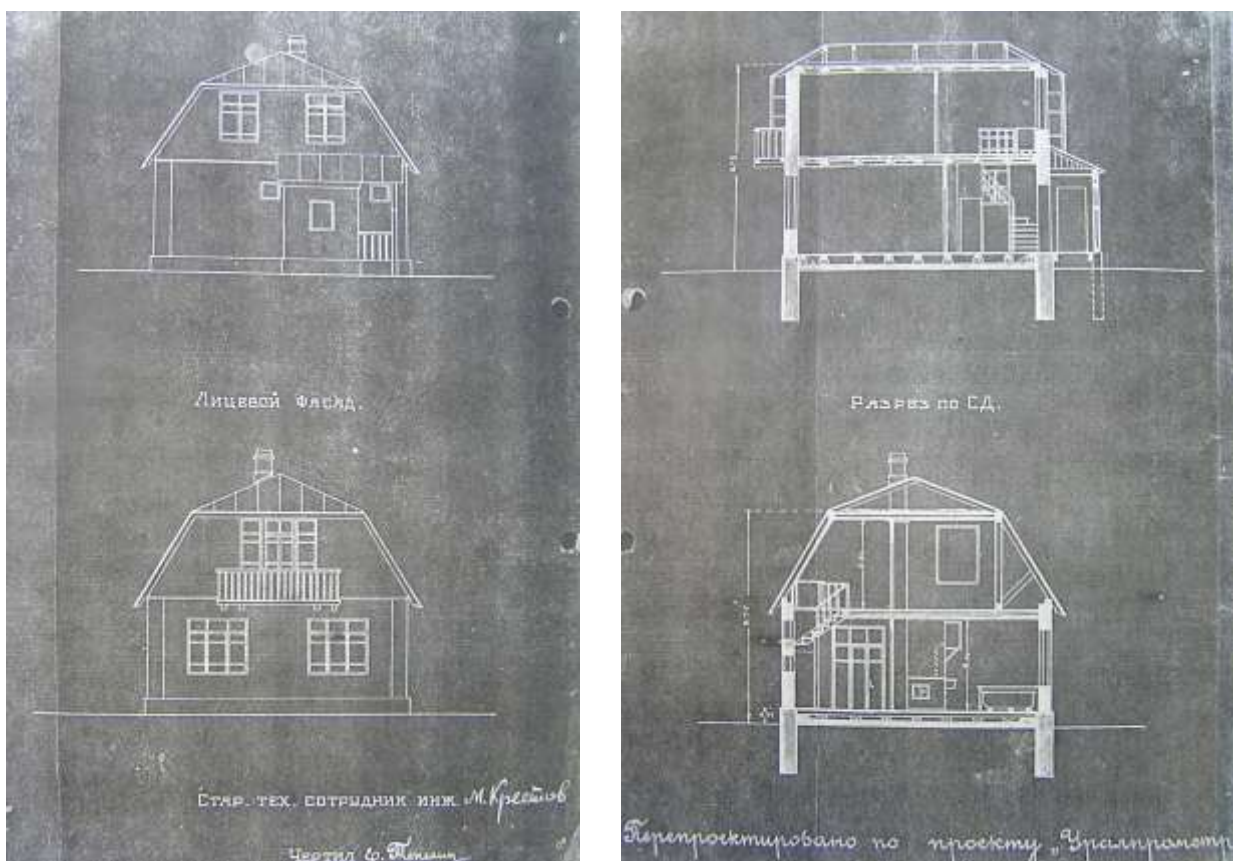
Илл.25. Жилой дом коттеджного типа усадебной застройки в г. Свердловске. Переработанный проект «Уралпромстроя». Фасады. Источник: Предоставил Л. Эррен
