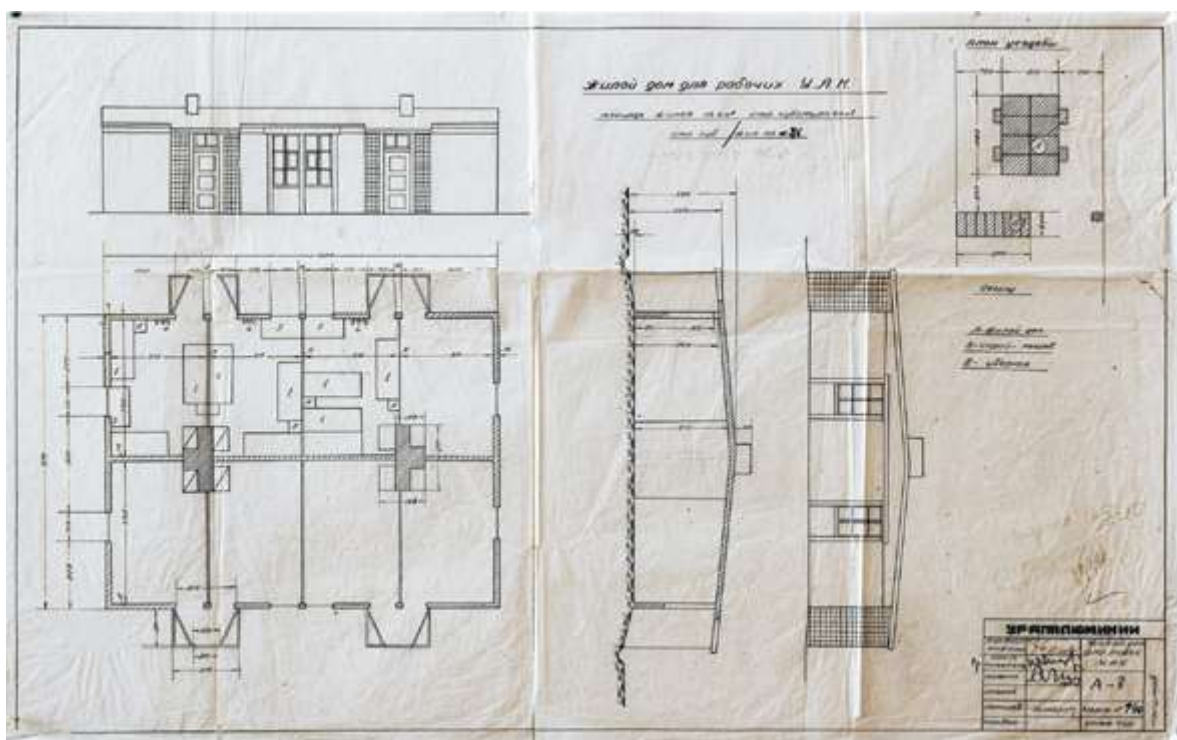
Илл.22. Проект каркасно-камышитового жилого дома А-8. «Уралалюминий» УАЗ, 1935-1940 гг.(Архив УАЗ-СУАЛ). Источник: Гаврилова С.И. Архитектура 1930-х годов Красногорского района г. Каменска-Уральского [Электронный ресурс] / С.И. Гаврилова //Архитектон: известия вузов.- 2009. -№3 (27). - Режим доступа: http://archvuz.ru/numbers/2009_3/ta1
