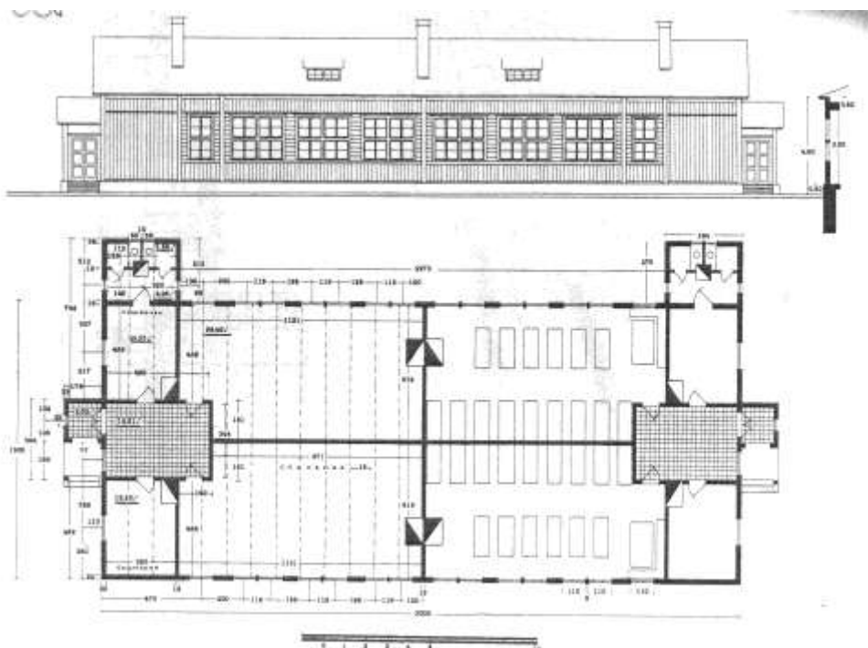
Илл. 7. Барак (одноэтажный, деревянный) на 50 человек со столовой. Проект. 1929. Источник: Проекты рабочих жилищ. Центральный банк коммунального хозяйства и жилищного строительства. М. 1929. – С.203.
