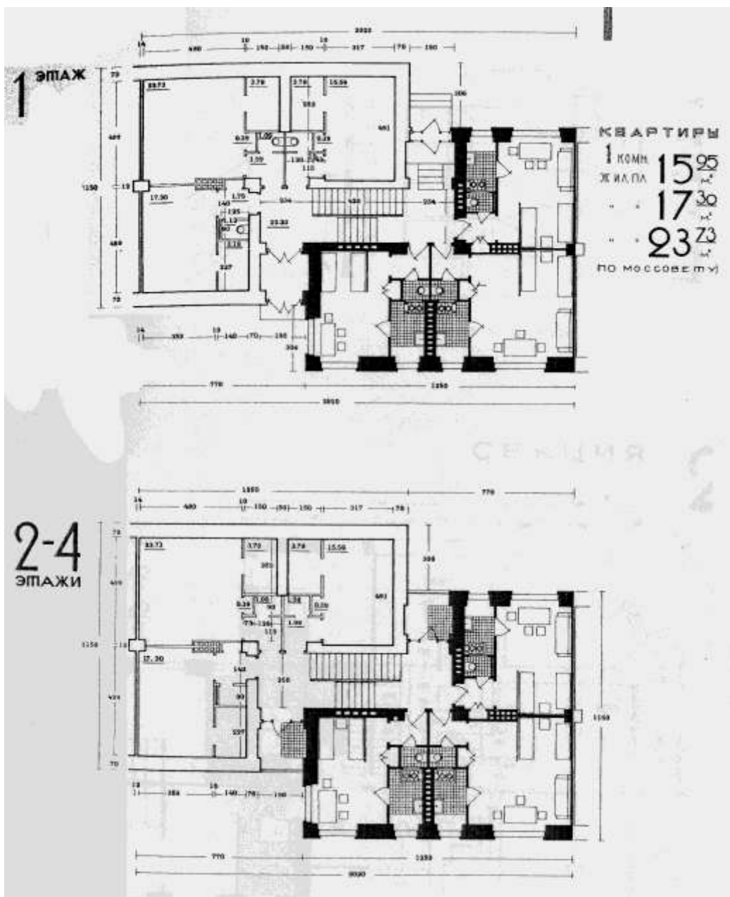
Илл.19. Секционный 3-4-х этажный каменный жилой дом, рассчитанный на покомнатно-посемейное заселение, рекомендуемый для массового строительства. 1929.
