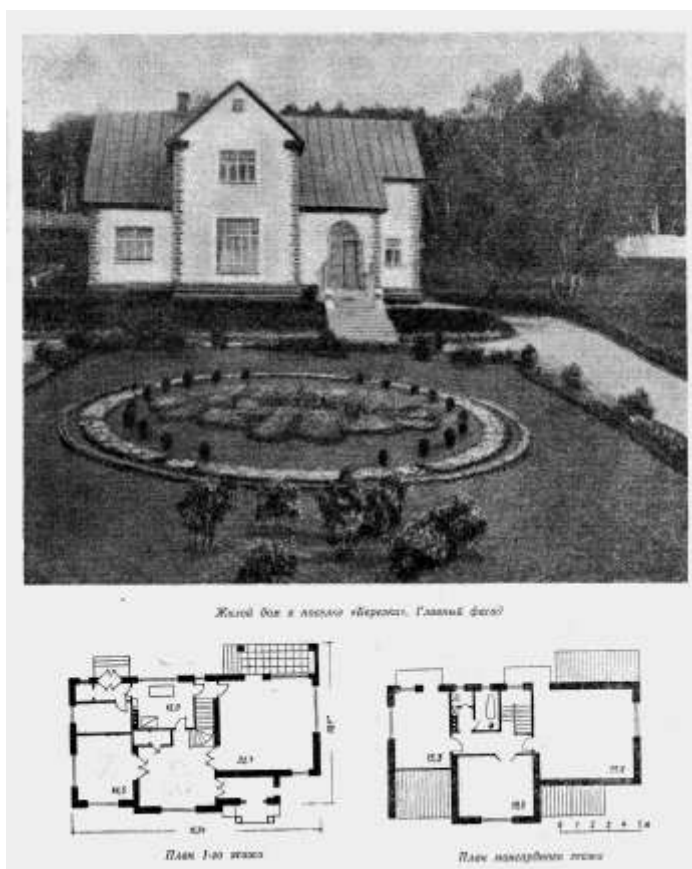
Илл.11. Соцгород Магнитогорск. Жилой дом в поселке «Березки». Фасад, планы. 1930-е гг. Источник: Шасс Ю. Архитектура жилого дома. Вып.1. Поселковое строительство 1918-1948 годов. Государственное издательство литературы по строительству и архитектуре. М. 1951. – 200 с., Таблица 25.
