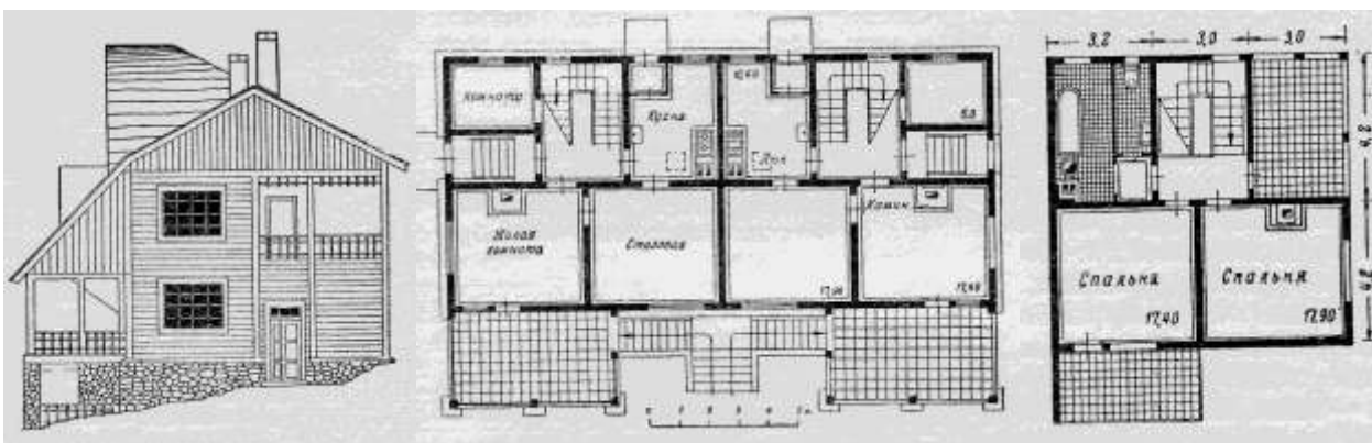
Илл. 16 Кузнецкстрой. Верхняя колония. 2-х квартирный каркасно-засыпной коттедж. Фасады. Планы. 1929.
