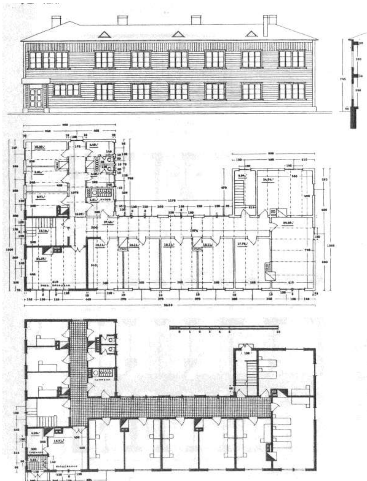
Илл. 5. Общежитие (2-х этажное, деревянное) на 40 человек. Проект. 1929. Источник: Проекты рабочих жилищ. Центральный банк коммунального хозяйства и жилищного строительства. М. 1929. – С.191.
