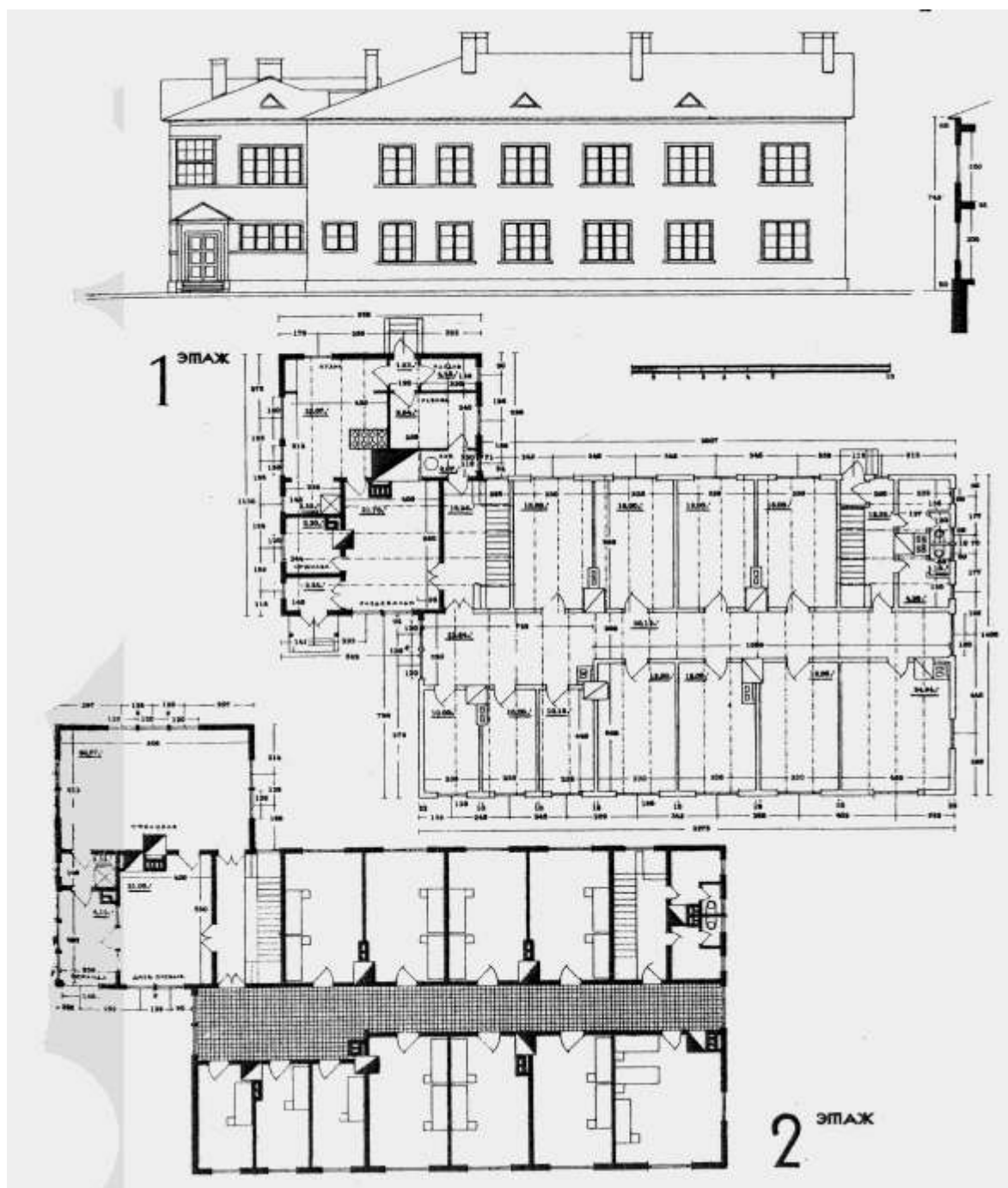
Илл. 6. Общежитие (2-х этажное, каменное) на 40 человек. Проект. 1929. Источник: Проекты рабочих жилищ. Центральный банк коммунального хозяйства и жилищного строительства. М. 1929. – С.193.
