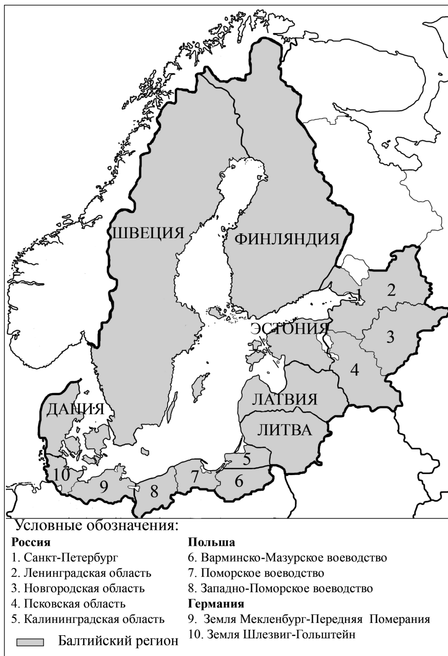
Рисунок 3. Балтийский регион в узком смысле
