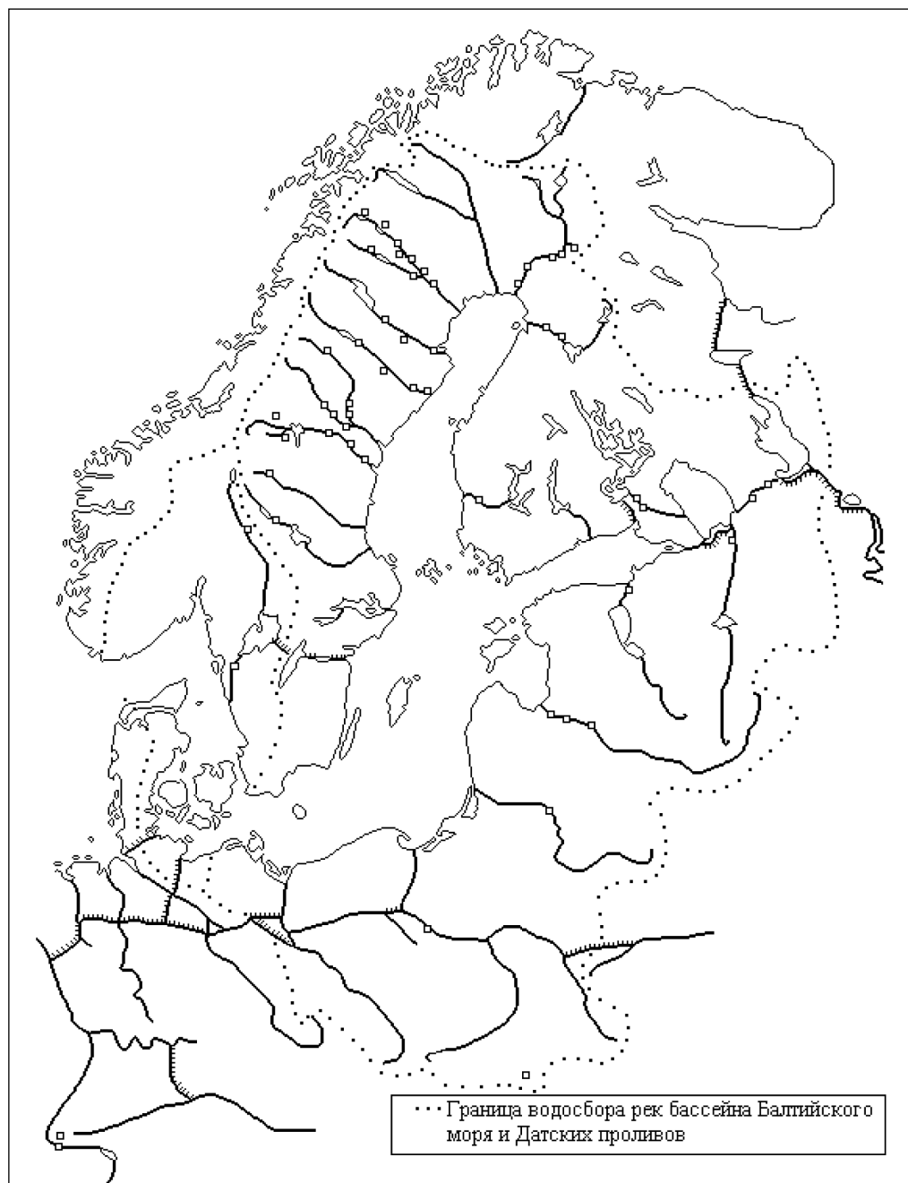
Рисунок 2. Бассейн Балтийского моря
