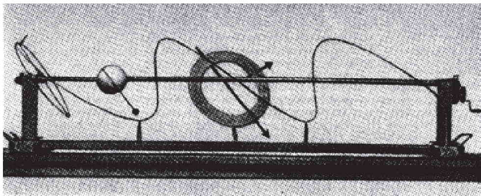
Рис. 4. Модель геликоидального движения Земли в Галактике, иллюстрирующая «солнечную гипотезу» проф. Д. Пиккарди
