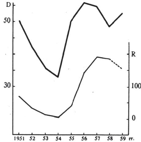
Рис. 2. Динамика экспериментов D (верхняя кривая) и солнечной деятельности – чисел Вольфа (нижняя кривая). Коэффициент корреляции равен 0,85 [по Д. Пиккарди]
