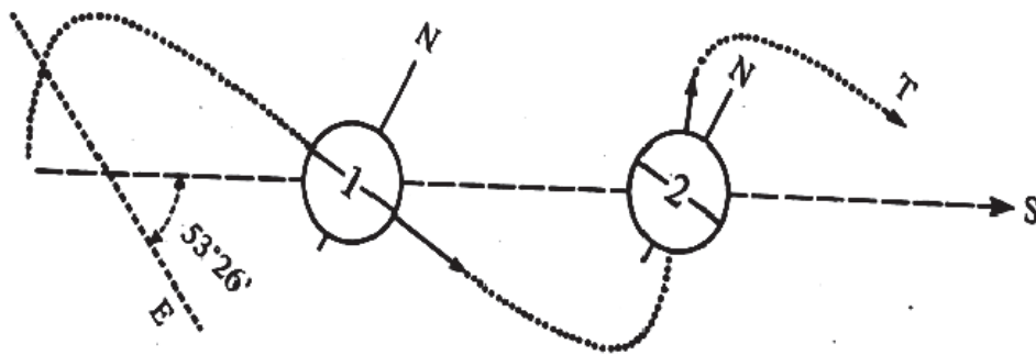
Рис. 3. Движение Земли в направлении центра Галактики: E – плоскость эклиптики в профиль, S – апекс Солнца, N – направление Северного полюса Земли, T – геликоидальное движение Земли [по Д. Пиккарди]
