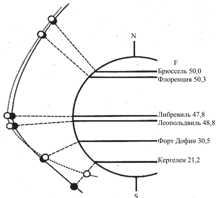
Рис. 5. Расположение основных лабораторий на земном шаре, где проводится изучение влияния солнечных вспышек на реакцию F .
