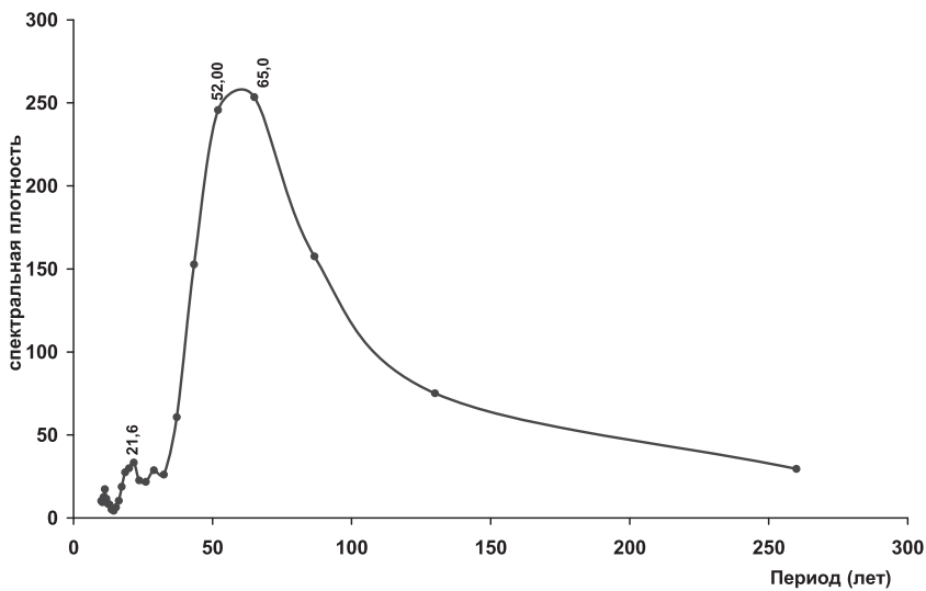
Рис. 42. Спектр Фурье (Италия)
