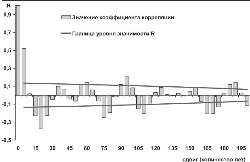
Рис. 38. Автокорреляционная функция «цивилизационного маятника» России
