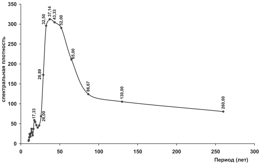
Рис. 39. Спектр Фурье (Россия)
