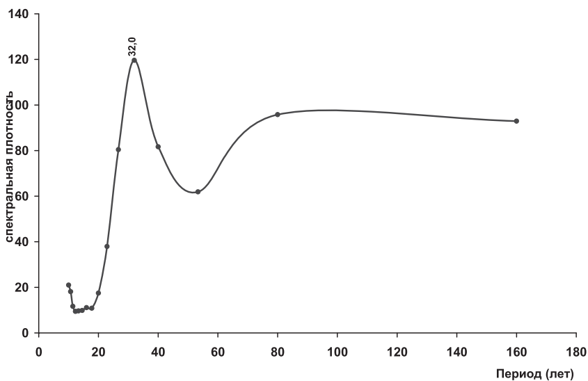
Рис. 48. Спектр Фурье (Япония)
