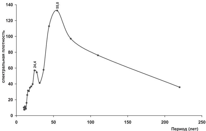
Рис. 49. Спектр Фурье (Бразилия)
