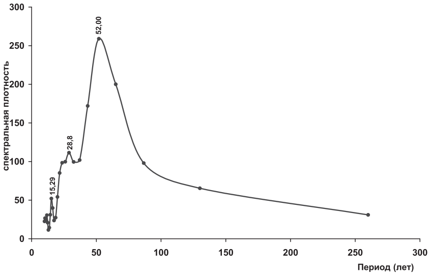
Рис. 43. Спектр Фурье (Германия)
