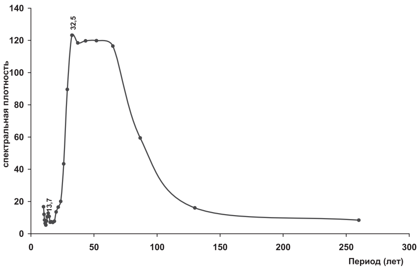
Рис. 44. Спектр Фурье (Великобритания)
