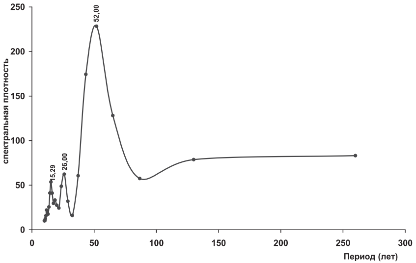
Рис. 46. Спектр Фурье (Китай)
